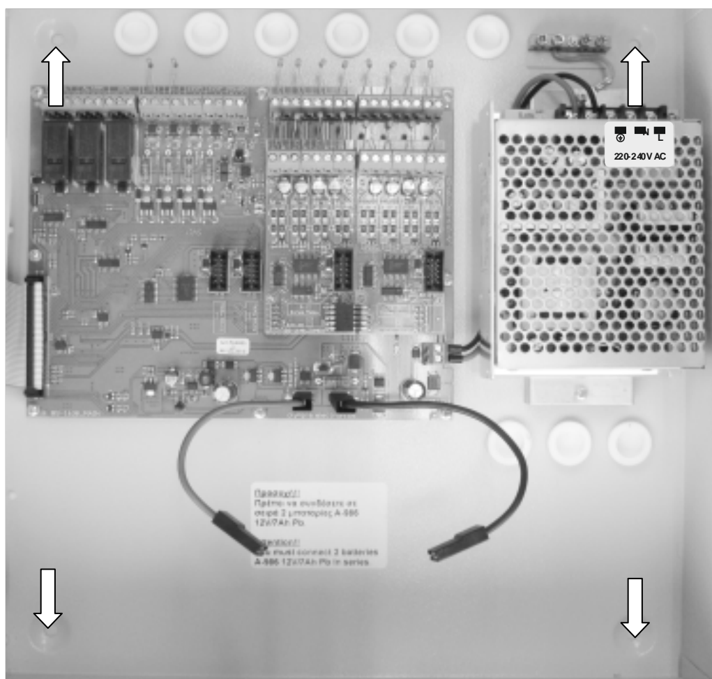
Εικόνα 4-1. Πίνακας ασφαλείας και υλικά στήριξης.
