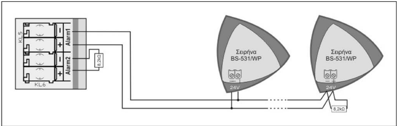
Σχήμα 4-8. Σύνδεση σειρήνων
