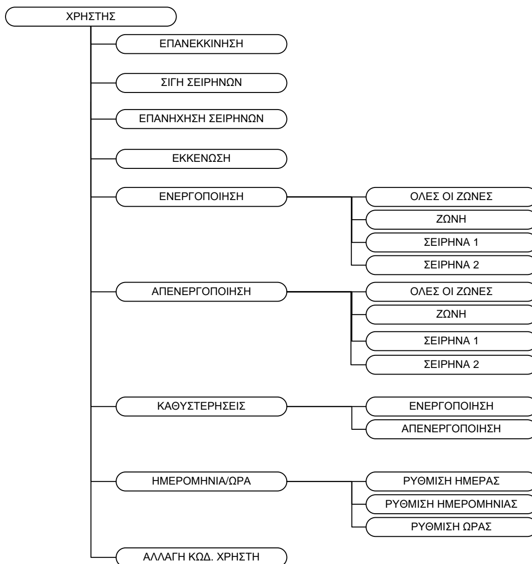
3-3. Δομή μενού
